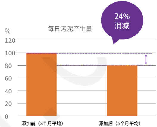
图-2 实验期间的污泥生产量
